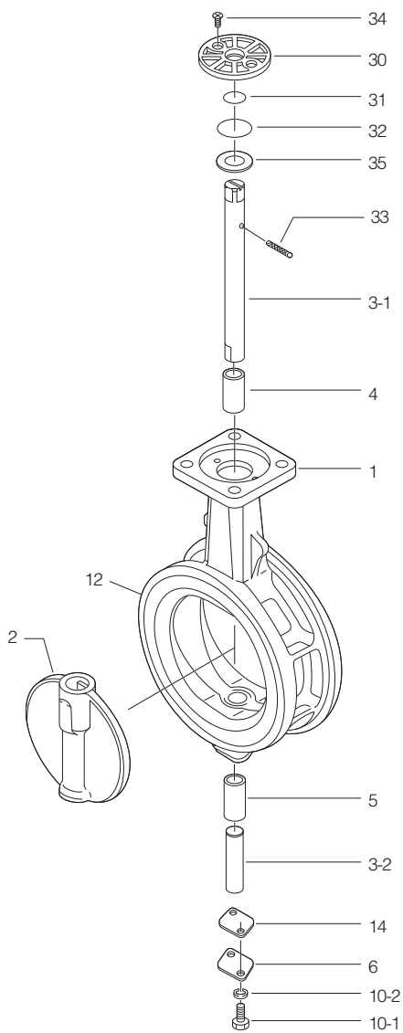
■732P本体部部品表 (50mm~300mm)
