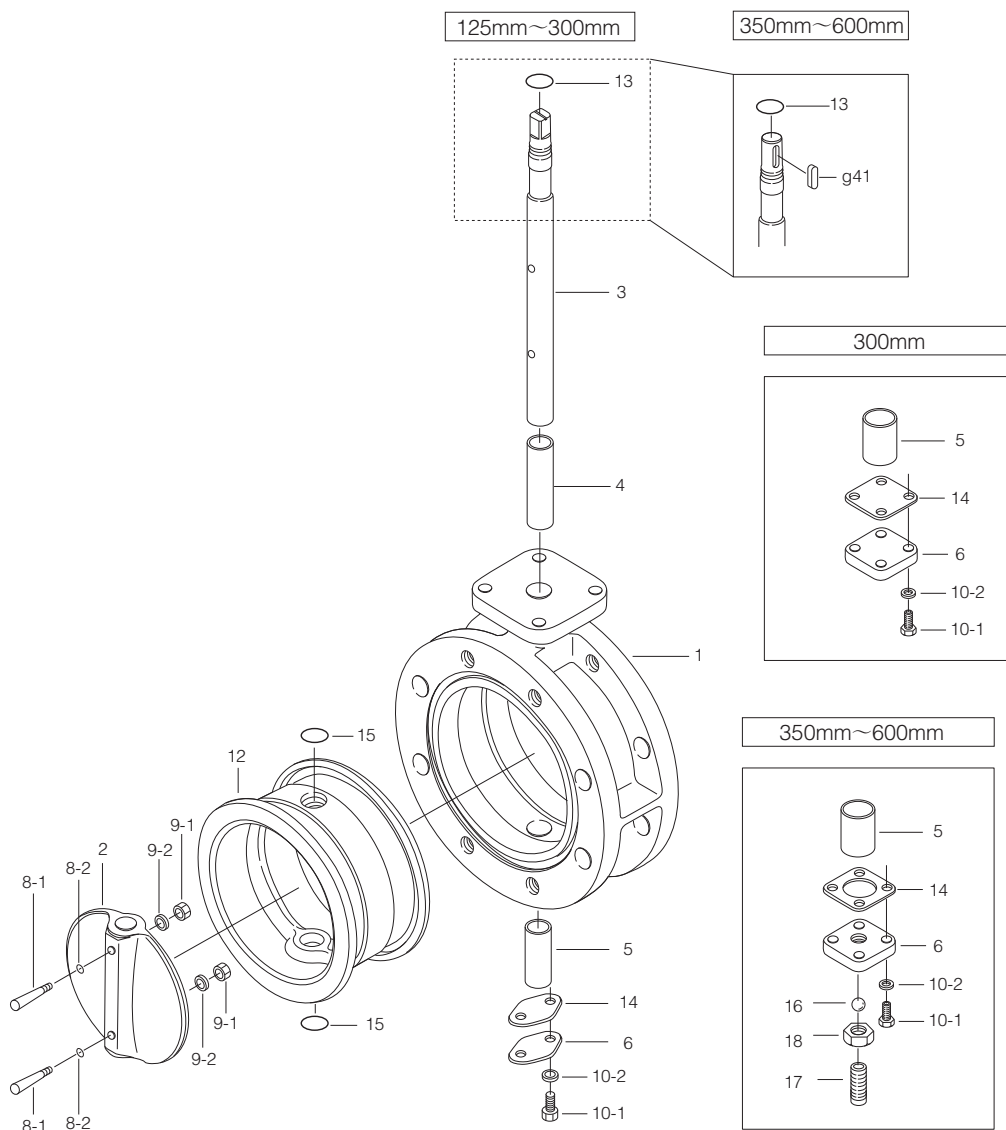
■722F本体部部品表 (125mm~300mm)
