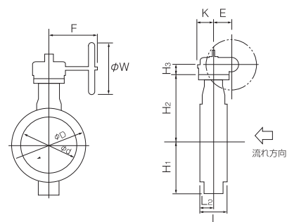
■ウォームギヤ式 304YA-2U (40～300mm)
