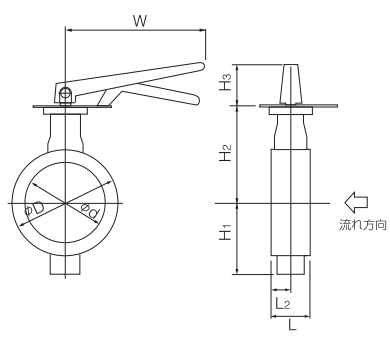
■ロックレバー式 302Y-1T (40~150mm)
