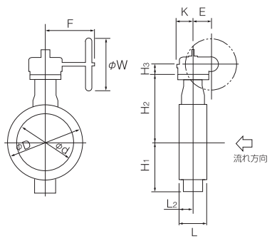
■ウォームギヤ式 302Y-2U (40~150mm)/302Y-2S (200mm)
