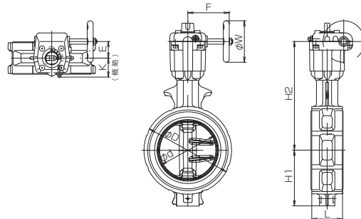
■ウォームギヤ式 700Z-2F
