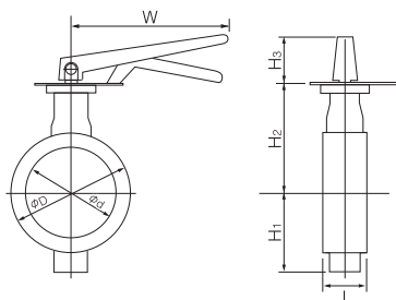
■ロックレバー式 700Z-1J(40～125mm) 700Z-1T(150mm)
