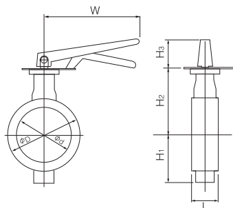
■ロックレバー式 701G-1T
