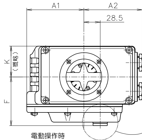
電動操作時
