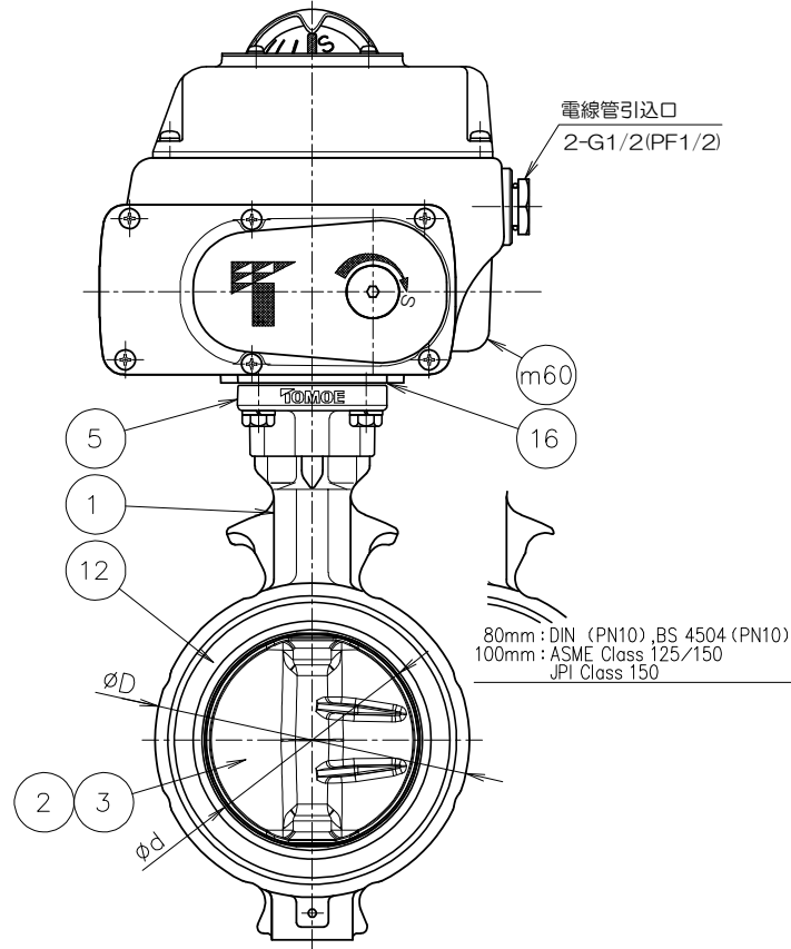
電動操作時
