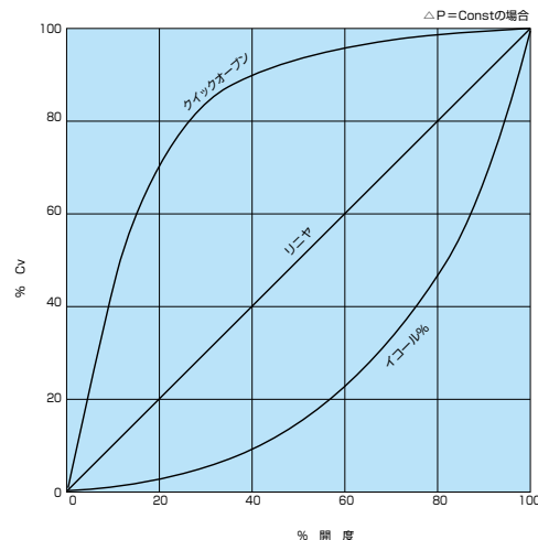
固有流量特性
