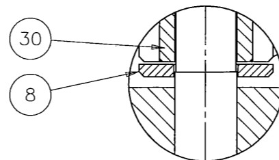
C 詳細図
