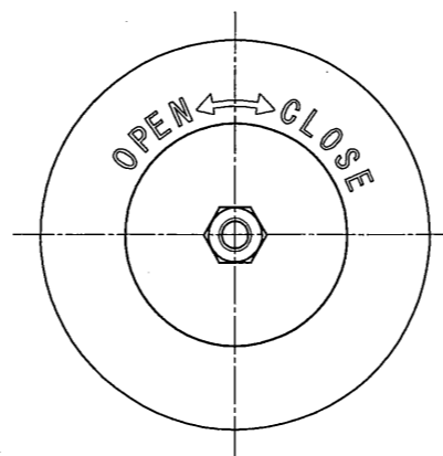
B 矢視図
