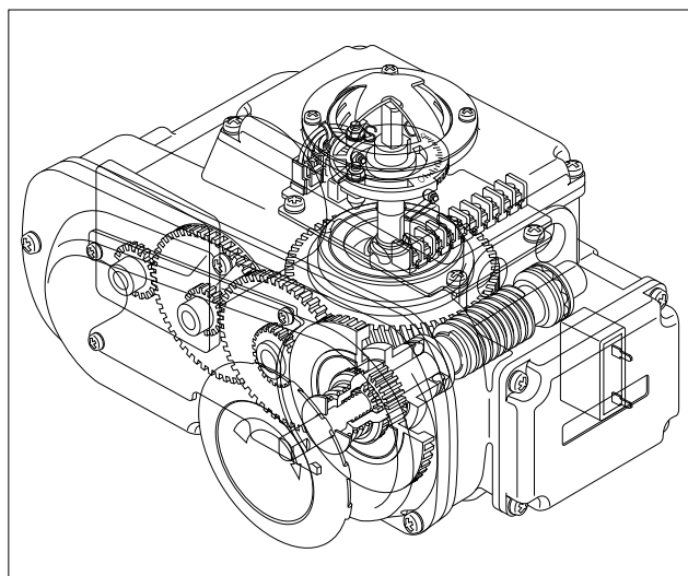
New ELMY 構造図
