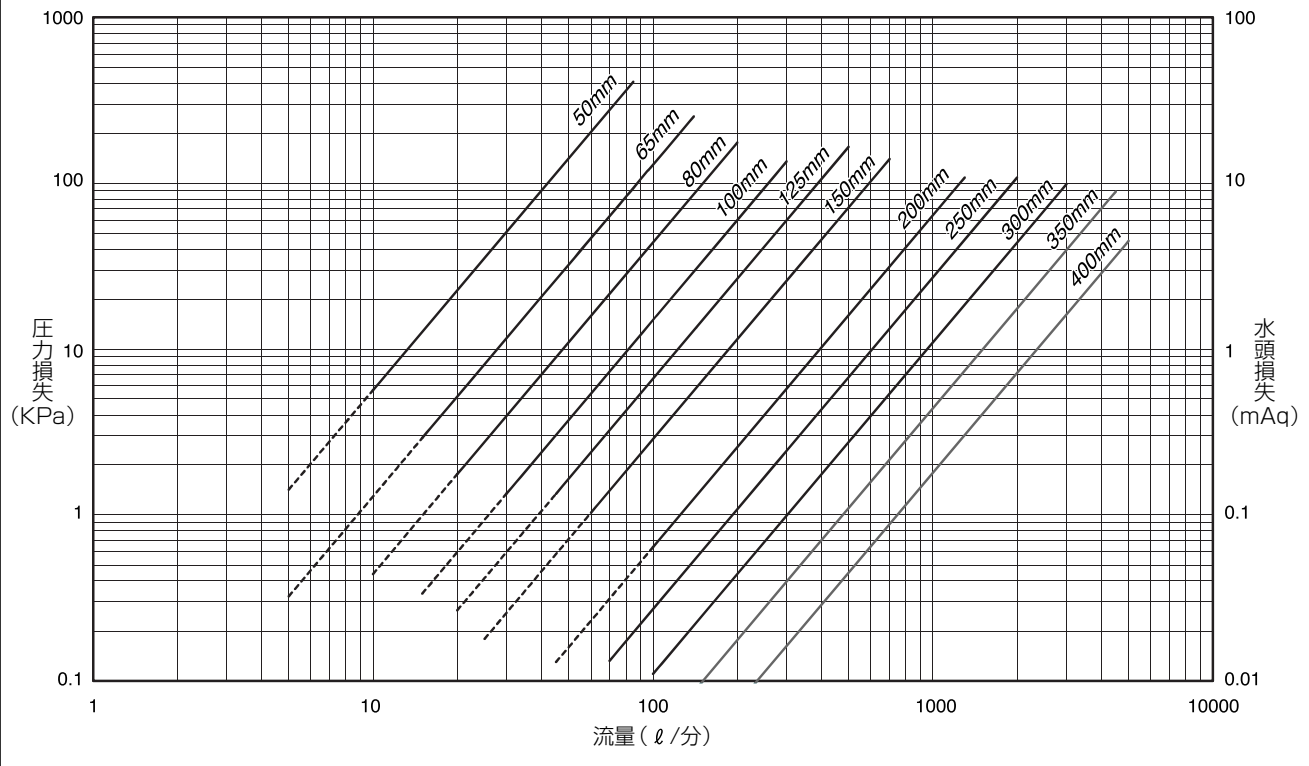
907H/908H 標準トルクスプリング圧力損失
