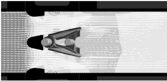
注)色は圧力分布を示します。赤色は高圧部、青色は低圧部です。矢印の大きさは流速の大きさを示します。 高圧 ←—————→ 低圧
