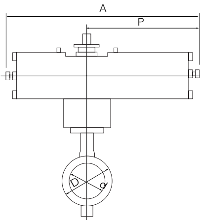
空気圧シリンダ(3K)取付け方向
