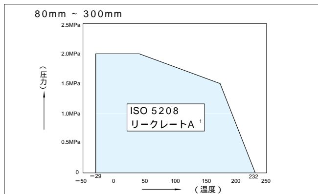
ISO 5208バルブの圧力試験
